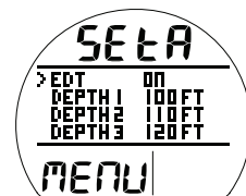
Fig. 103 - SET A MENU
